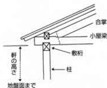
洋 小 屋
