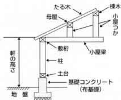
和 小 屋
