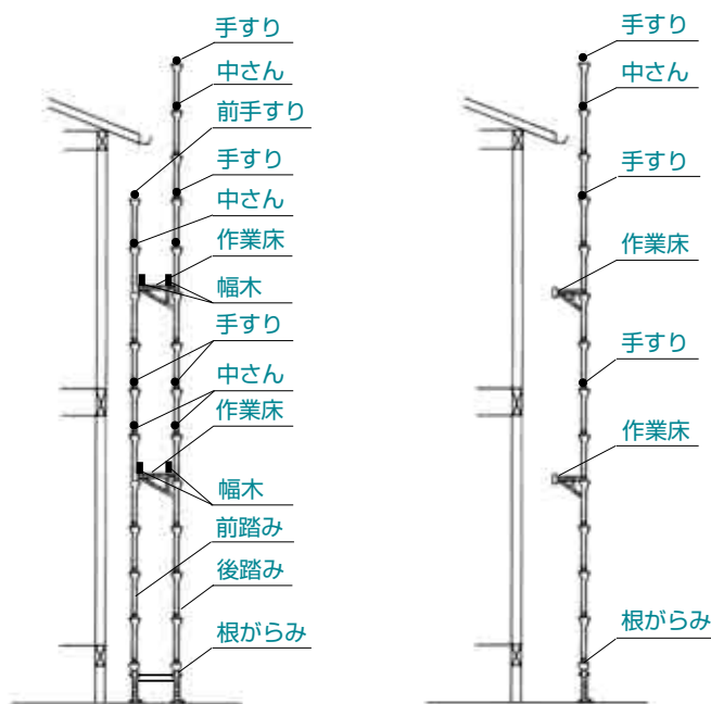
二側足場の例
